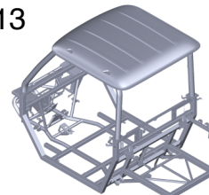
FRAME AND ROOF STRUCTURE STRUTTURA TELAIO E TETTO
